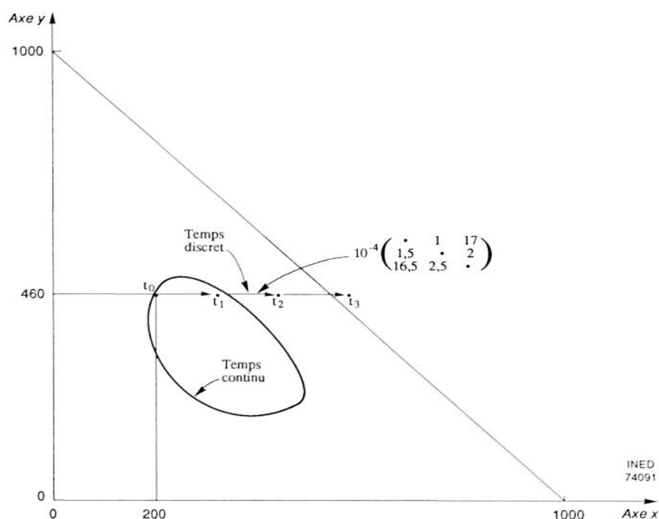
Figure 3. – Variation des populations y_n (cf. y(t) ) en fonction de x_n (cf. x(t) ) lorsque la trajectoire, en temps discret, sort du domaine de définition des populations ( y_3 ) tandis qu'en temps continu, cette trajectoire est toujours dans ce domaine.
