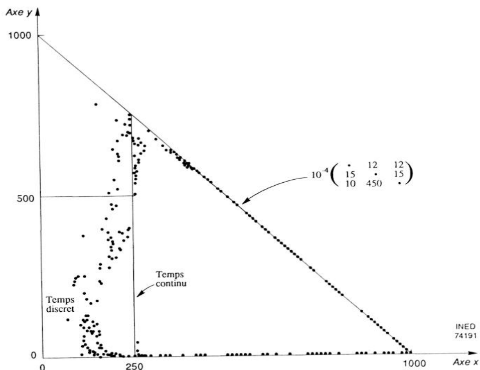
Figure 4. – Variation des populations y_n (cf. y(t) ) en fonction de x_n (cf. x(t) ), lorsque la trajectoire, en temps discret, devient « chaotique » tandis qu'elle reste bien définie en temps continu.
