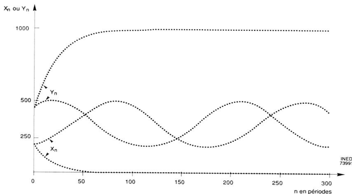
Figure 2. – Variation des populations x_n et y_n en fonction de la période intercensitaire n dans les deux cas décrits dans la figure 1.
