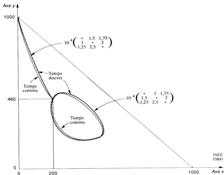
Figure 1. – Variation des populations y_n (cf. y(t) ) en fonction de x_n (cf. x(t) ) dans le cas d'une trajectoire fermée et dans le cas d'une trajectoire tendant vers le point (0,1000), partant de populations initiales identiques (200, 460, 340).
