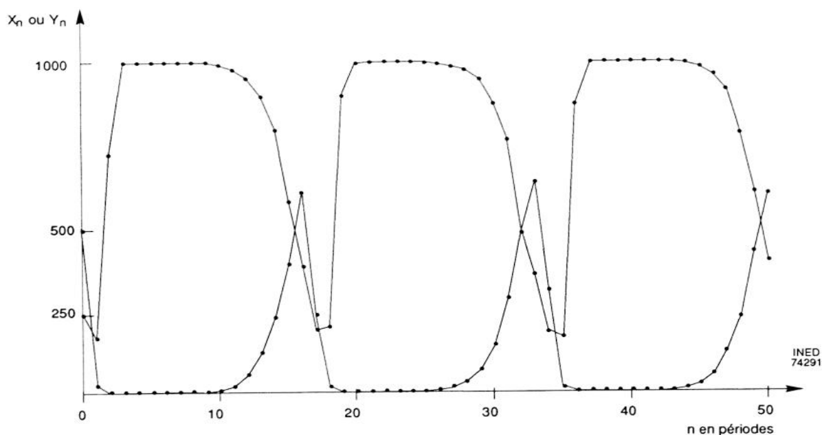
Figure 5. – Variation des populations x_n et y_n en fonction de la période intercensitaire n dans le cas « chaotique » décrit dans la figure 4.
